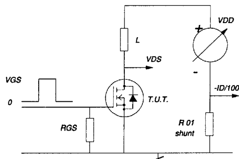
Fig. 16. Avalanche energy test circuit.
